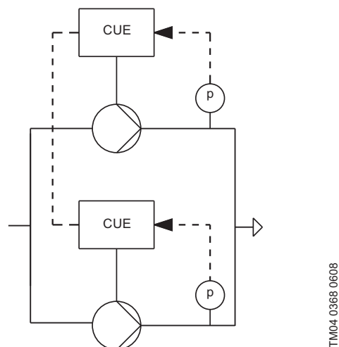
Рис. 26 Два насоса, соединённых параллельно и регулируемых через GENIbus
