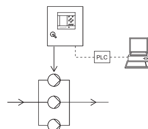
Рис. 29 Разомкнутый контур (внешний контроллер)
