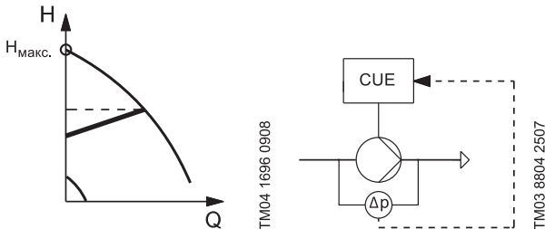
Рис. 31 Пропорциональный перепад давления, обновление H_{\max}
