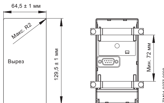
Рис. 55 Монтаж шкафа, размеры выреза
