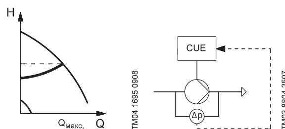
Рис. 30 Перепад давления, параболическая кривая
